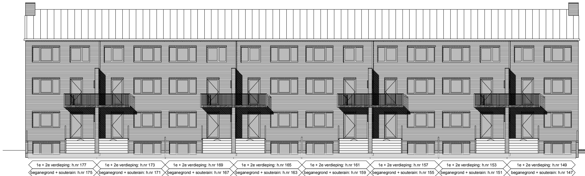
Zuidgevel
