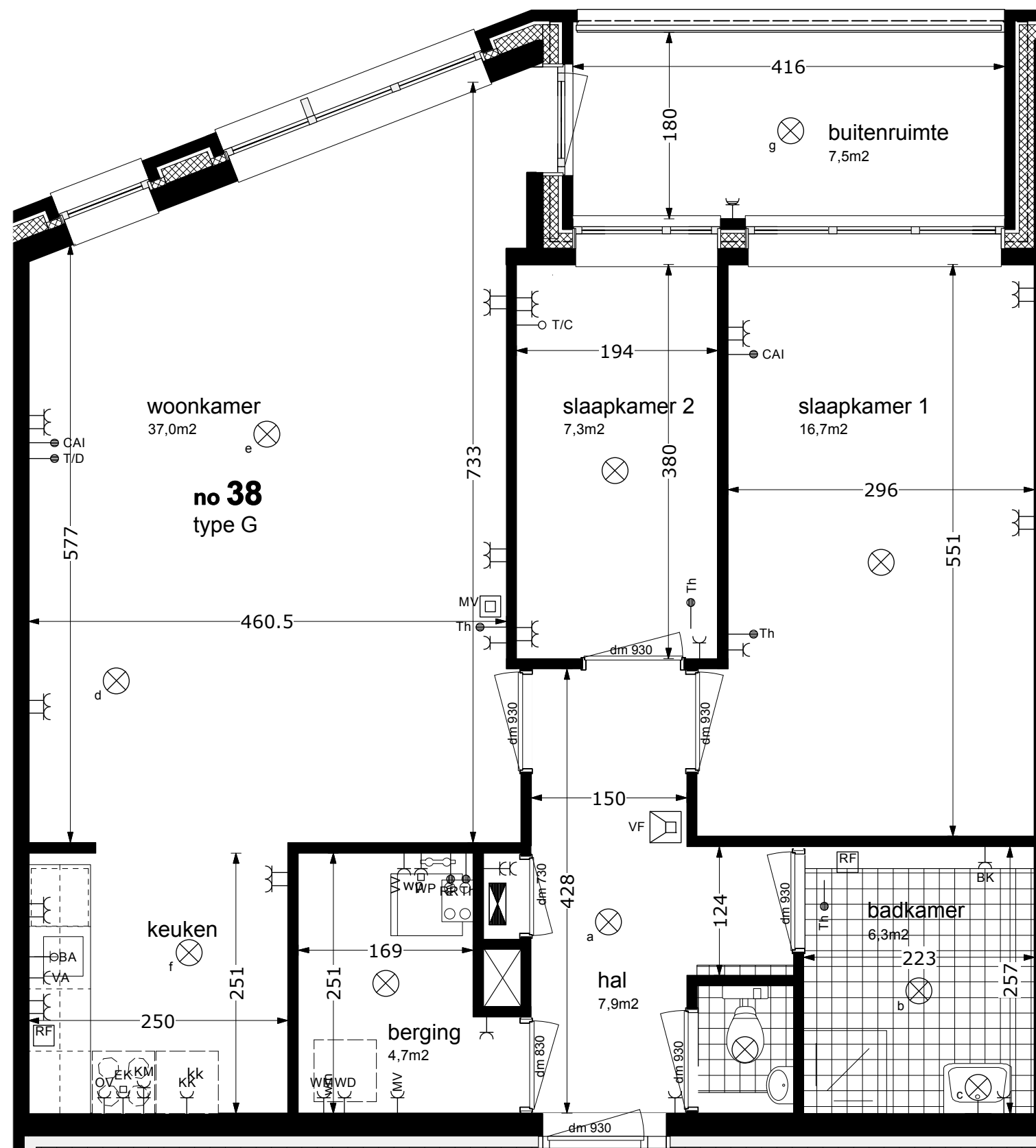
Plattegrond woning (2e verdieping)
