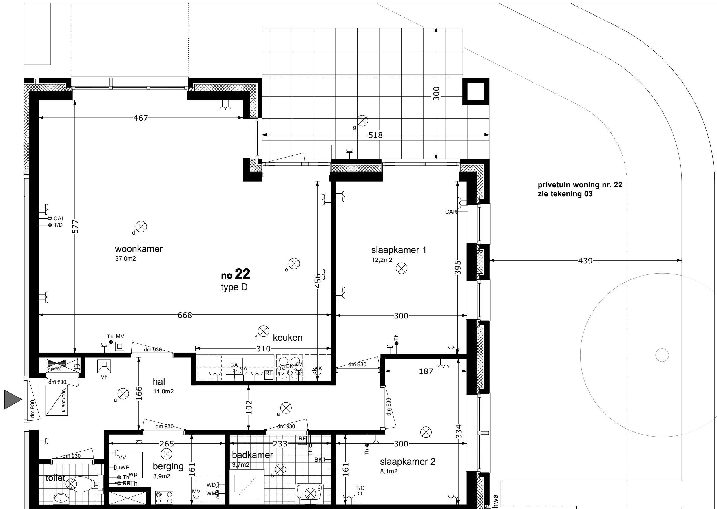
Plattegrond woning (begane grond)
