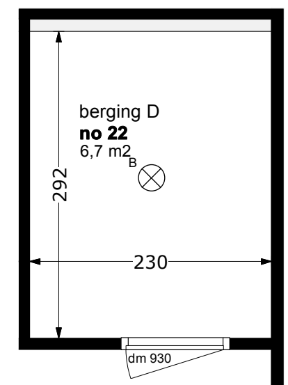
Plattegrond berging begane grond
