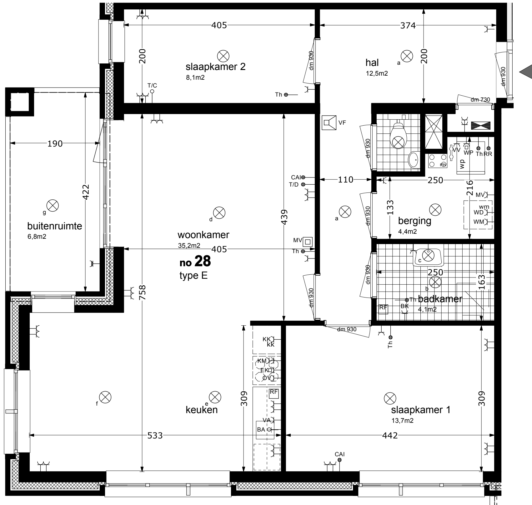
Plattegrond woning (1e verdieping)
