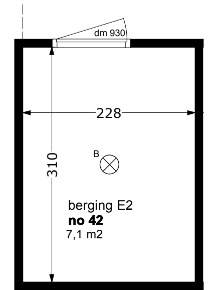
Plattegrond berging begane grond
