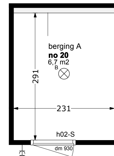
Plattegrond berging begane grond
