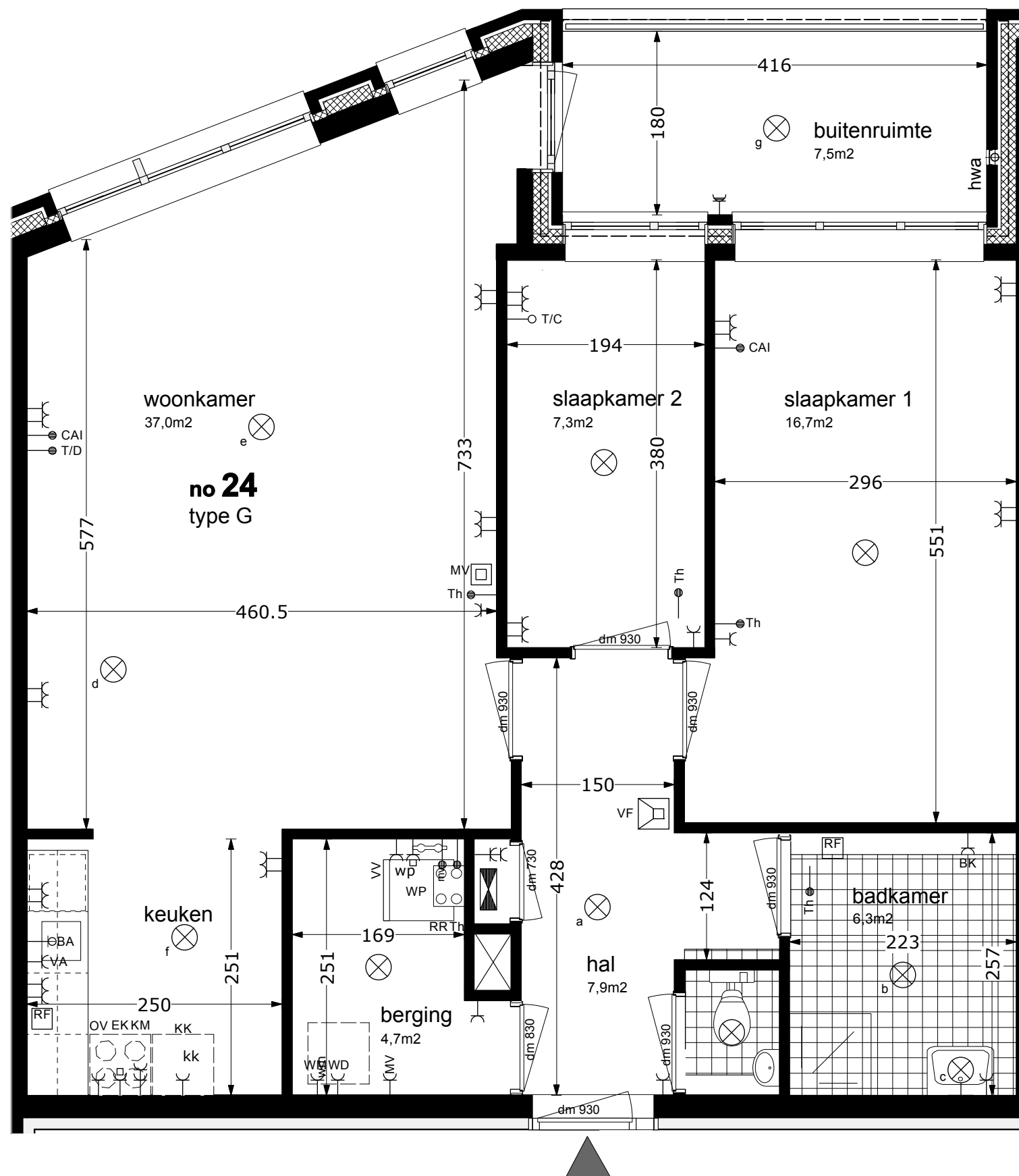
Plattegrond woning (1e verdieping)
