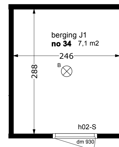
Plattegrond berging begane grond
