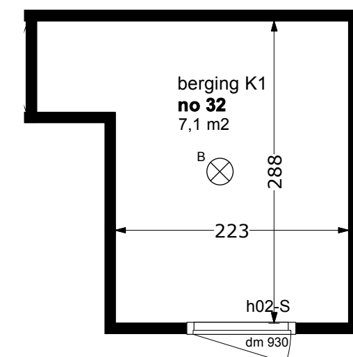
Plattegrond berging begane grond
